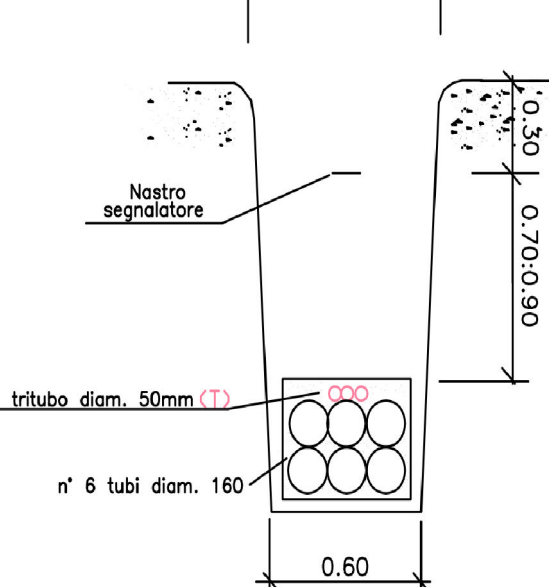
Sezione tipo su marciapiede
