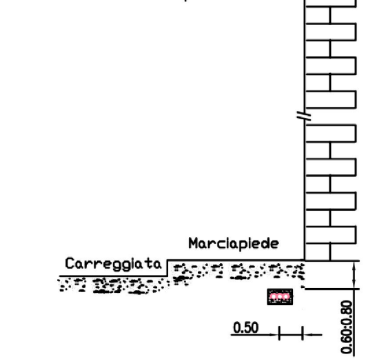
Sezione tipo su marciapiede
