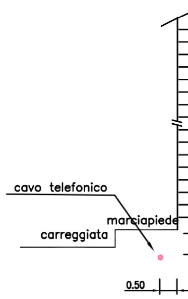
Sezione scavo su carreggiata
