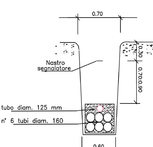
Sezione tipo di attraversamento
